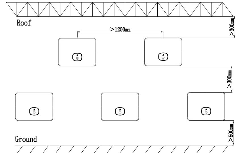
Abb 5.3 Installationsschema mehrerer Wechselrichter
